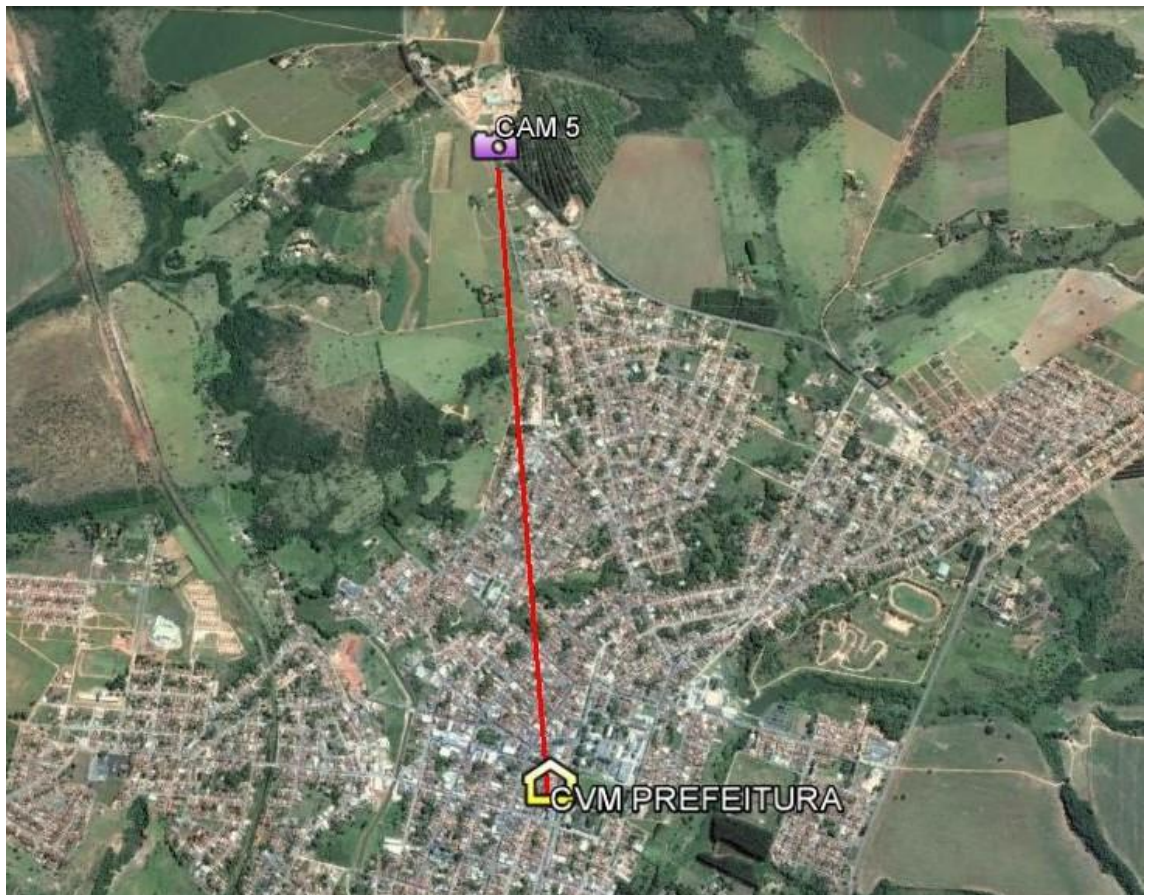
Figura 02: 1 ponto de câmera 01 Link de Rádio Ponto a Ponto 01 Central de vídeo monitoramento (CVM amarela)
