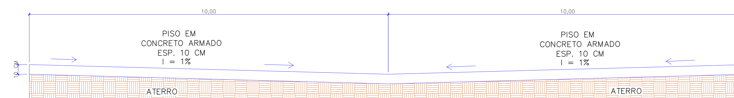
SECÇÃO TRANSVERSAL PISO ARMADO
